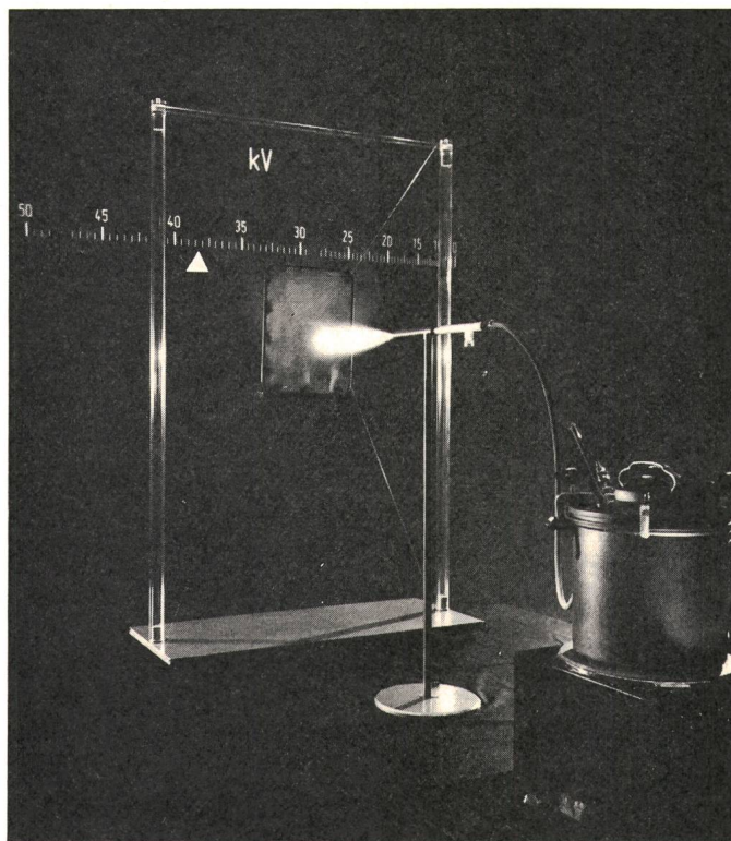
Fig. 18 Wasserdampfelektrizität
