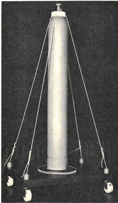
Fig. 19 Isolierte Druckluftflasche
