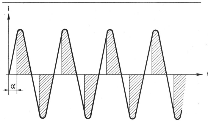
Fig. 2 Phasenanschnitt-Steuerung
