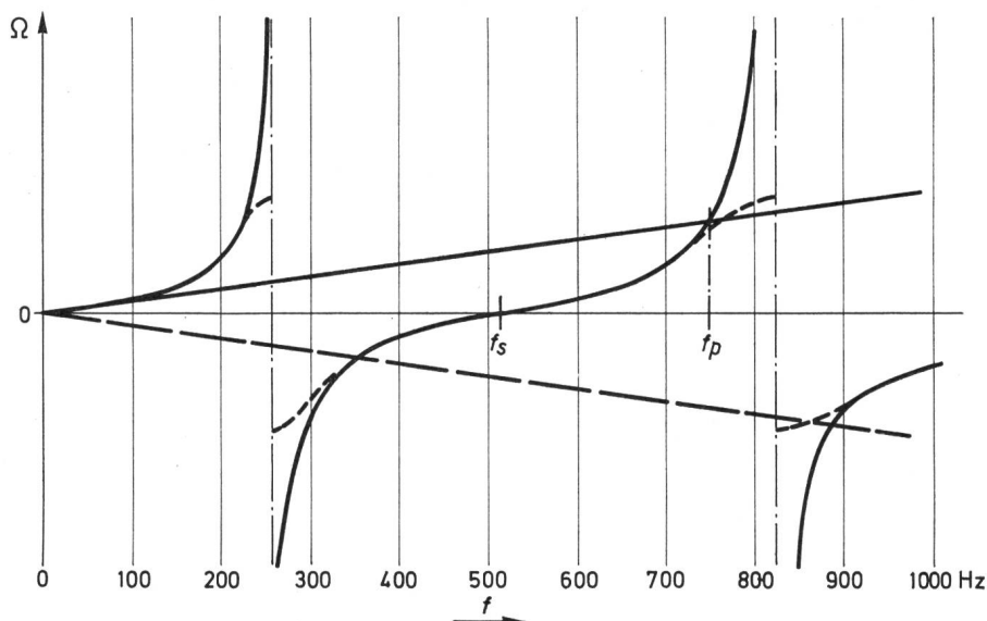
Fig. 9 Einfluss eines gesperrten Kondensators auf die Netz-Reaktanz – Reaktanzverlauf der Schaltung nach Fig. 8 f_s Serieresonanz-Frequenz f_p Parallelresonanz-Frequenz
