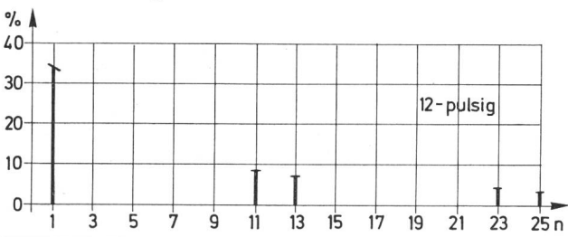
Fig. 6 Durch Zusammenschaltung von zwei symmetrischen Drehstrom-Brücken heben sich weitere Oberschwingungen bestimmter Ordnungszahlen auf (in Fig. die 5., 7., 17. und 19. Harmonische) n Ordnungszahl
