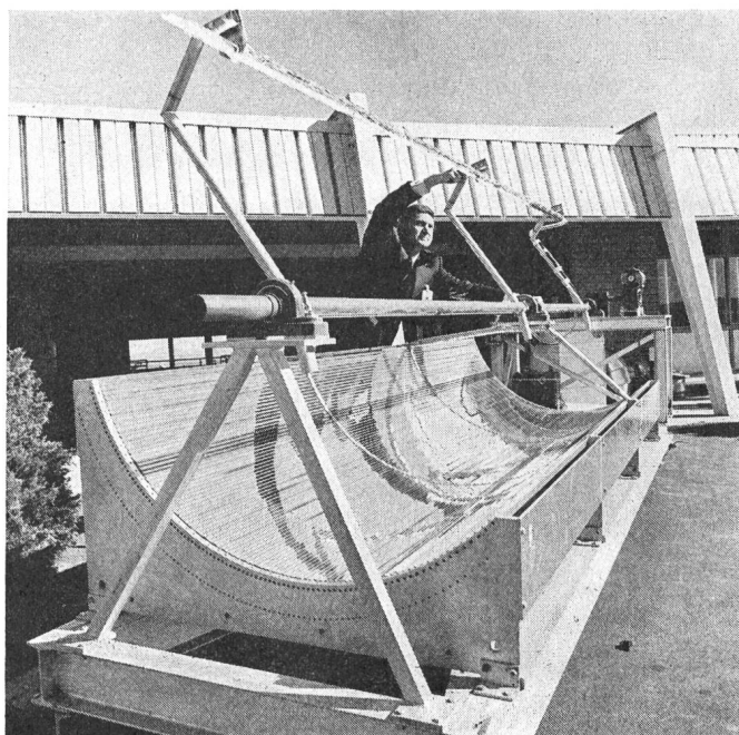
Fig. 4 Versuchsmodell des Sonnenspiegels
