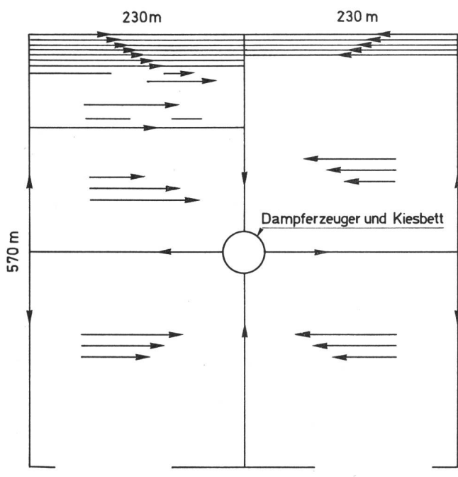
Fig. 2 Grundriss einer Einheit mit 125 beweglichen Wärmeabsorptionsrohren in vier Quadranten
