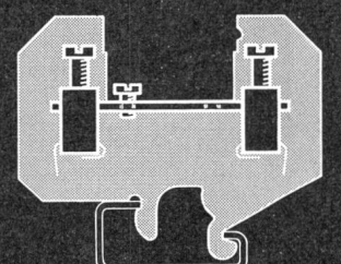
Querverbindungsklemme
