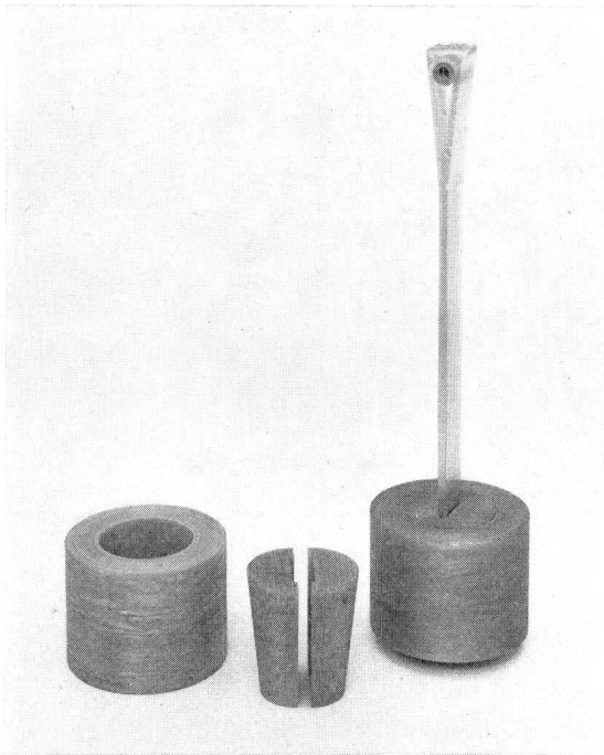
Fig. 13 300 mm lange Prüfstanze mit Armaturen aus GFK
