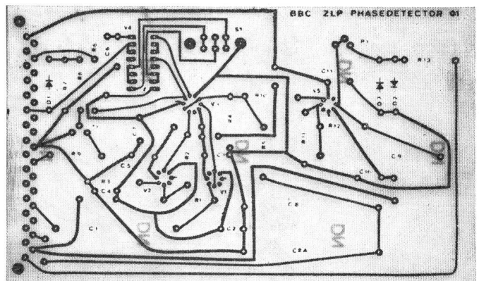
Fig. 14 Printplatte aus GFK
