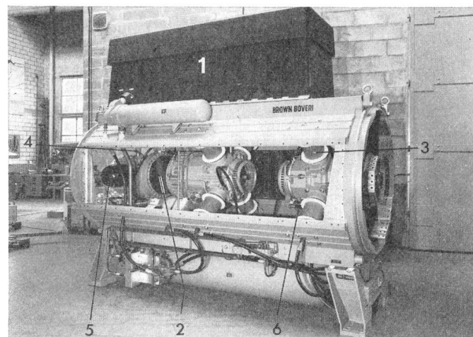
Fig. 9 Druckluft Generatorschalter
