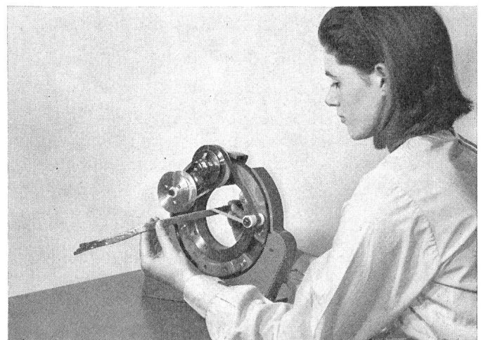
Fig. 2 Aufwickeln von Glasfasergewebeband auf einen Kupferleiter
