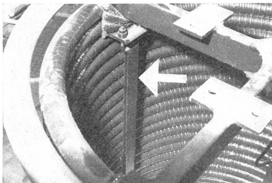
Fig. 11 Zugstange in einer Trägerfrequenzsperre
