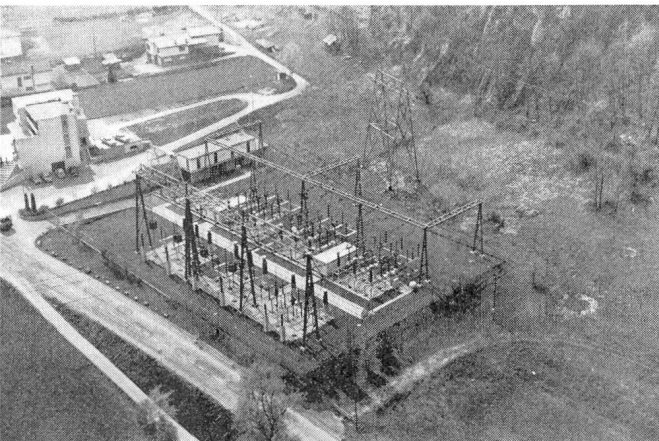
Fig. 6 220-kV-Schaltanlage Gorduno
