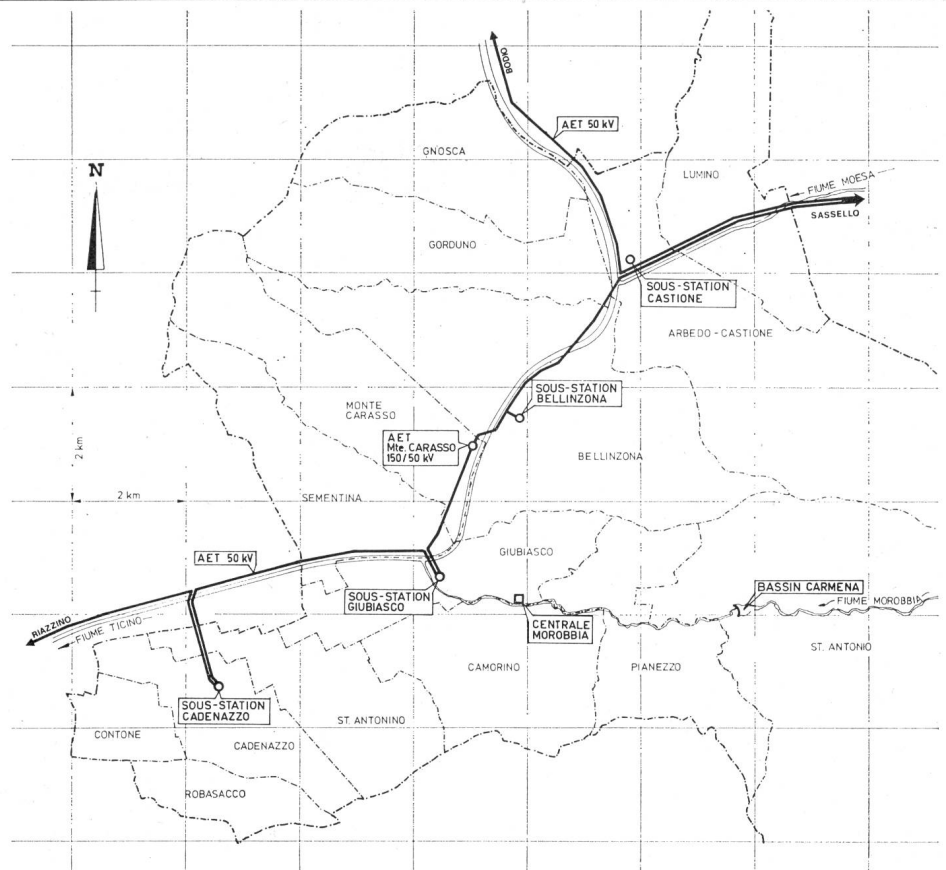
Fig. 6 Zone alimentée et sous-stations 50/16 kV
