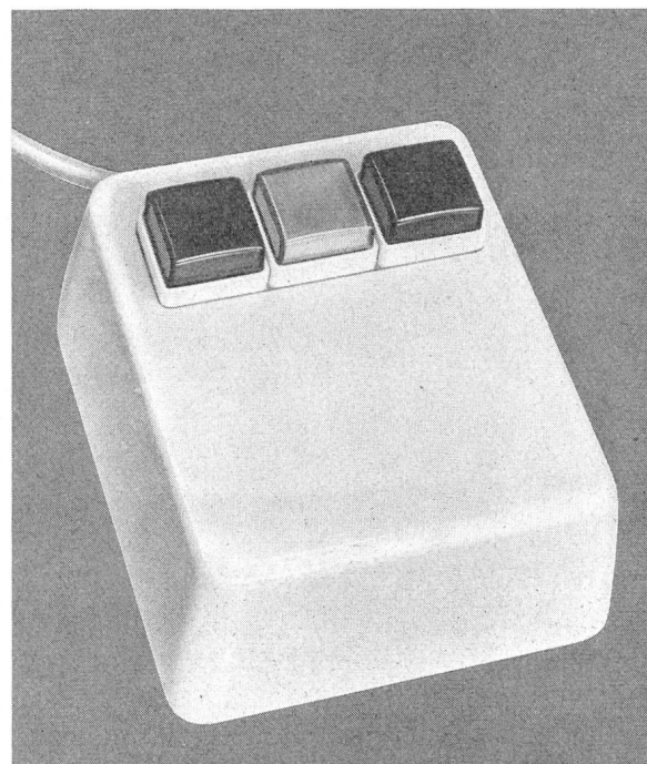
Tischstation mit drei Leuchtdruckschaltern und Summer, mit Kabel und Anschlussrosette
