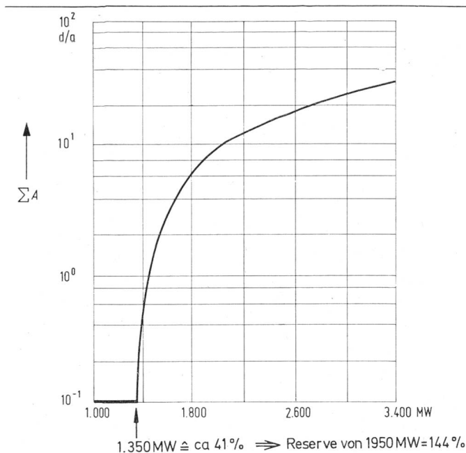
Fig. 5 Abhängigkeit der Ausfallerwartung von der Netzspitzenlast für das Beispiel von drei Maschinen
