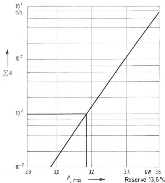
Fig. 7 Abhängigkeit der Ausfallerwartung von der Netzspitzenlast für das Beispiel mit 32 Maschinen von 50 bis 400 MW Leistung
