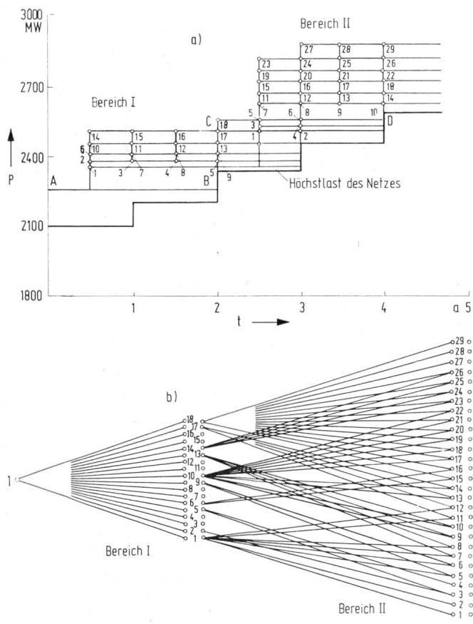
Fig. 2 Bestimmung der Ausbauplanung a Definitionsbereiche für zu planende neue Anlagen b Topologische Darstellung der Definitionsbereiche und ihre logischen Verknüpfungen
