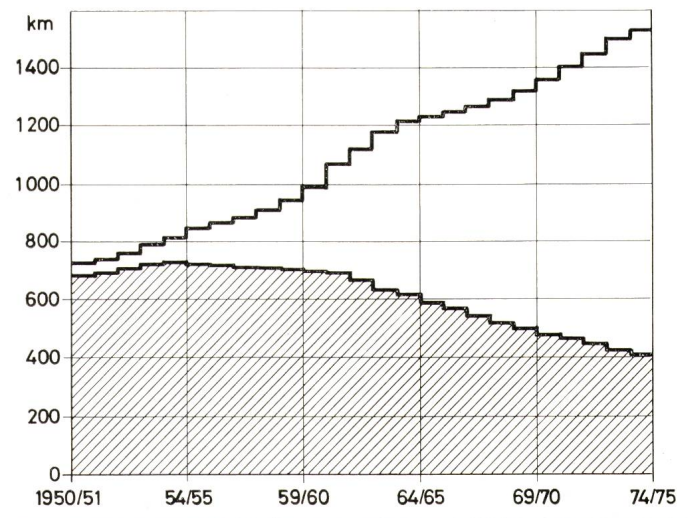
Fig. 3 Niederspannungsnetz (totale Länge der Freileitungen und Kabel)
