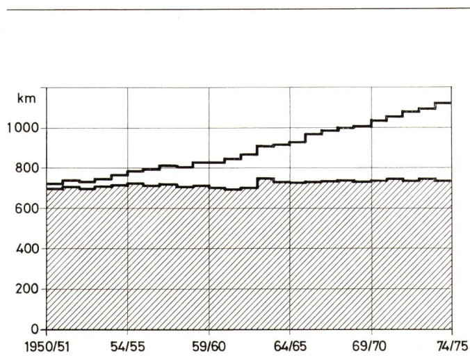
Fig. 2 16-kV-Hochspannungsnetz
