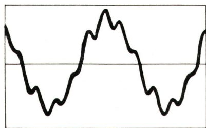
Fig. 3 Verzerrte Netzspannung durch Resonanz bei 350 Hz (7. Oberwelle)
