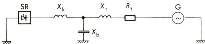
Fig. 6 Einphasiges Ersatzschaltbild von Fig. 5 bei 50 Hz ( m = 1 ) X_t, R_t Netzimpedanz
