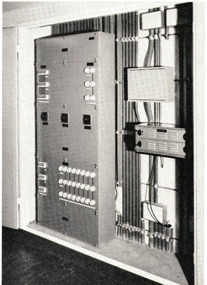
Fig. 2 Stockwerkverteiltabelleau mit Hauptschaltern, Leitungsschutzschaltern und Schmelzsicherungen
