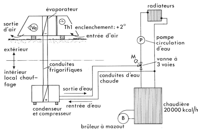
Fig. 1 Pompe à chaleur air-eau associée avec installation existante au mazout
