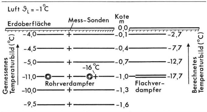
Fig. 1 Vergleich berechneter und gemessener Temperaturverteilung bei Wärmeentnahme aus dem Erdreich Mittelwert der Wärmeentnahmeleistung 4 kW/160 m 2
