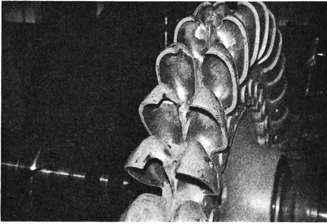
Fig. 1 Kraftwerk Oberrickenbach Peltonturbine 2380 PS vor der Erneuerung
