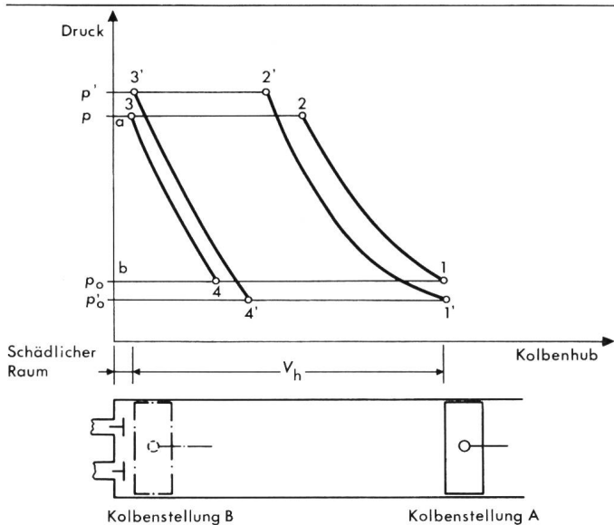
Fig. 2 Druckzyklus im Kompressor
