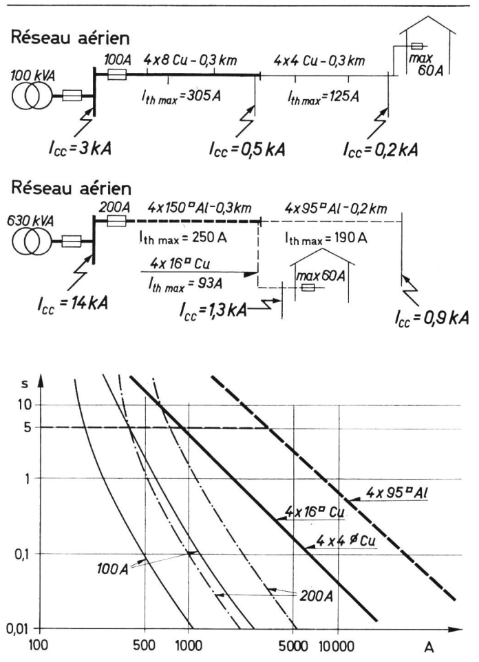
Fig. 2 Protection des «déseccionnements» traits gras: Durée admissible des court-circuits (en secondes) traits fins: Caractéristiques des fusibles (VDE 660 rapide)
