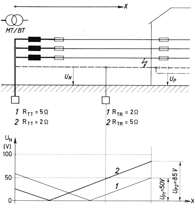
Fig. 3 Tensions entre neutre et terre X distance comptée à partir de la station transformatrice MT/BT
