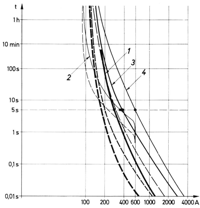
Fig. 5 Caractéristiques de fusion/déclenchement
