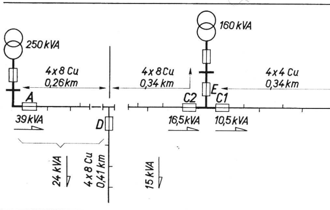
Fig. 6 Protection d'un réseau aérien BT après construction d'une nouvelle station transformatrice
