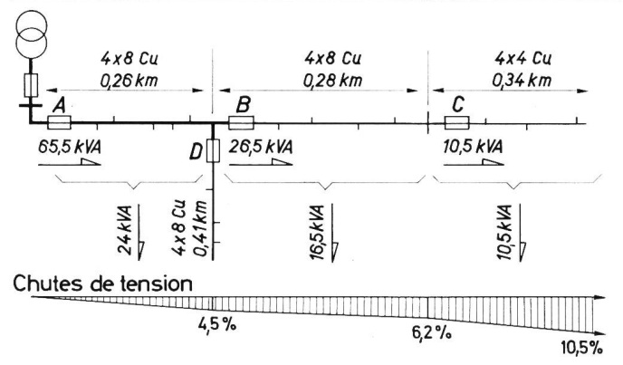
Fig. 4 Protection d'un réseau BT aérien
