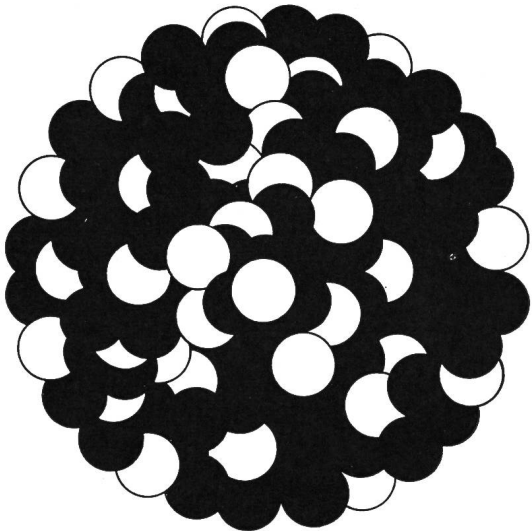
Uran-Atomkern
