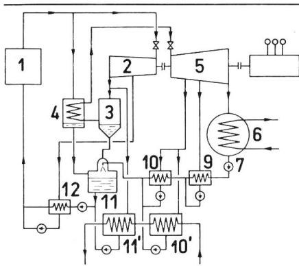
Fig. 6 Anlagenschema einer Kernkraftanlage mit Abgabe von Heizwärme aus Anzapfdampf
