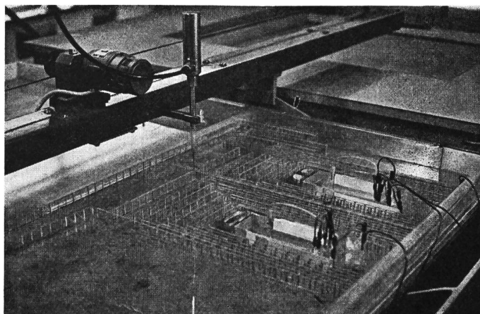
Fig. 7 Feldbild für die Dimensionierung einer Gleichspannungsisolation \pm 500 kV (USA)
