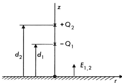
Fig. 1 Wolkendipol mit den Ladungszentren -Q_1 und +Q_2
