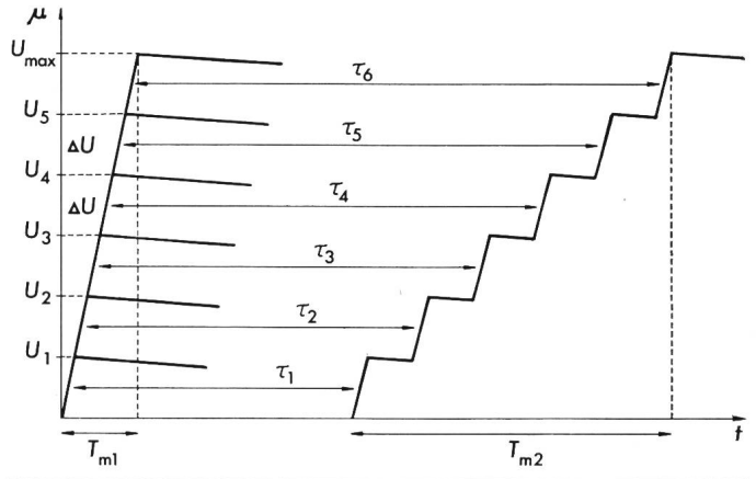
Fig. 6 Calcul de l'amortissement et de la déformation d'une onde de tension par découpage en échelons de tension T_{m1} temps de montée initial T_{m2} temps de montée final \tau_{1,2,...} temps de propagation de chaque échelon de tension \Delta U échelon de tension
