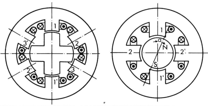
Fig. 1 (à gauche) Moteur réluctant triphasé, 12 pas par tour
