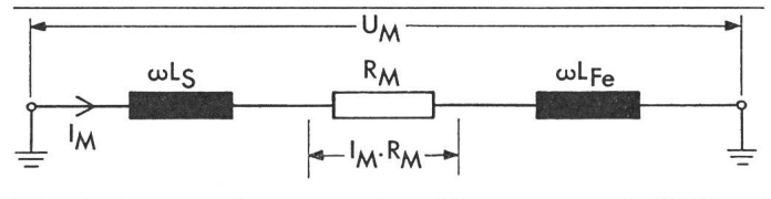
Fig. 3 Ersatzschaltbild einer Kabelhülle mit metallischem Kabelmantel und Bewehrung aus Bandeisen
