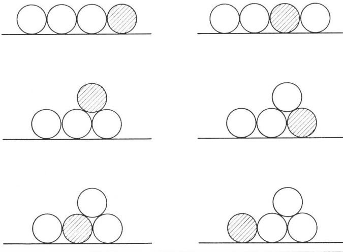
Fig. 2 Verlegungsmöglichkeiten eines Einleitersystems mit Nulleiter
