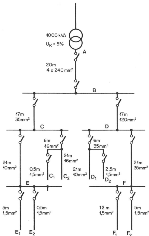
Fig. 1 Prinzipschema einer Industrieverteilung
