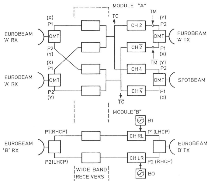
Fig. 4 OTS-Antennen und -Umsetzer
