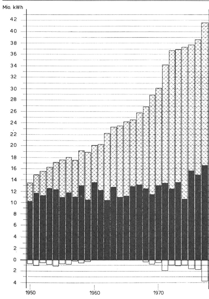
Fig. 6 Energie-Diagramm ▨ Energiebezug von KW Brusio ■ Eigenerzeugung □ Energieabgabe an KW Brusio
