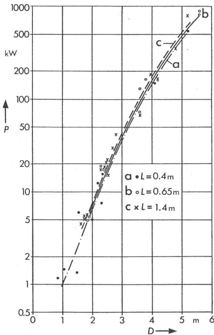
Fig. 1 Gesamte Ventilationsverluste P in Funktion der Statorbohrung D n^* = 300 \text{ U/min} Die Kurven umfassen a L = 0,3 \dots 0,5 \text{ m} b L = 0,53 \dots 0,8 \text{ m} c L = 1,0 \dots 1,8 \text{ m}
