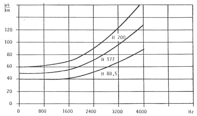
Fig. 6 Typischer Verlauf der Gruppenlaufzeit pro km von pupinisierten Leitungen
