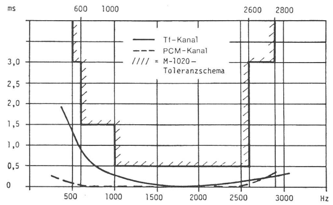
Fig. 8 Typischer Verlauf der Gruppenlaufzeitverzerrung bezogen auf das Minimum im Vergleich zur M-1020-Toleranzgrenze
