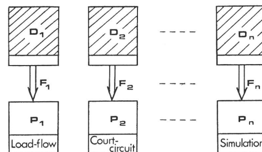
Fig. 1 Interaction données-programmes
