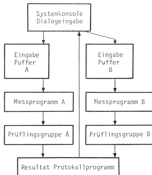
Fig. 5 Messdatenflussdiagramm
