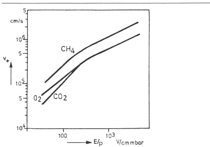
Fig. 10 Driftgeschwindigkeit der positiven Ionen in ihren Ursprungsgasen in Abhängigkeit von E/p [4]
