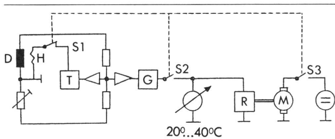
Fig. 1 Prinzipschaltbild eines Thermographiegerätes mit Kontaktsonde
