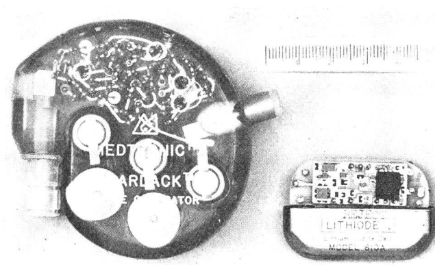
Fig. 8 Grössenvergleich (cm-Skala) eines Bedarfsschrittmachers mit diskreter Schaltung mit einem modernen Schrittmacher in Hybridschaltung sowie mit einer Lithiumjodid-Batterie
