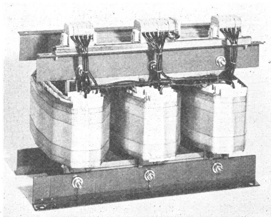
Bandgewickelter Dreiphasen-Transformator 25 kVA
