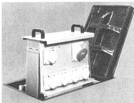
Befahrbarer Elektrans
