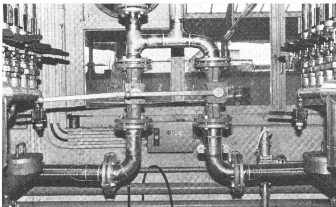
Rohrbegleitheizung mit Wärmekabel
