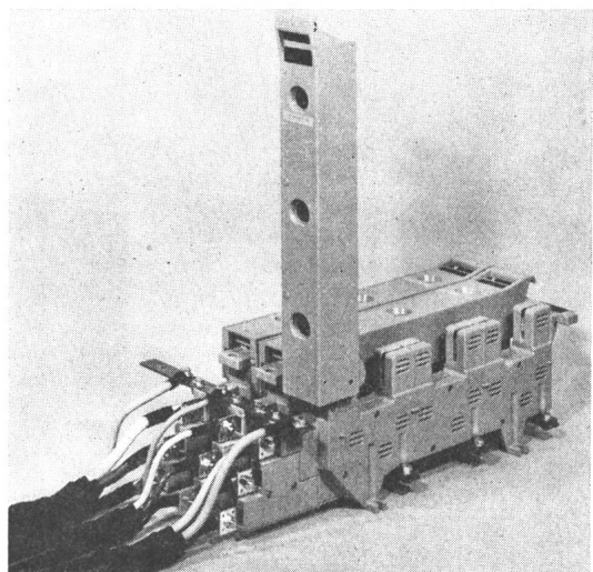
3polige Lasttrennsicherung Typ 2 V
