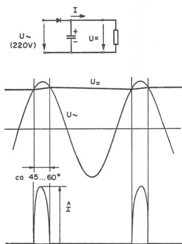
Fig. 1 Grundsätzliches Schema, Spannungen und Strom des Speiseteils eines Fernsehempfängers
