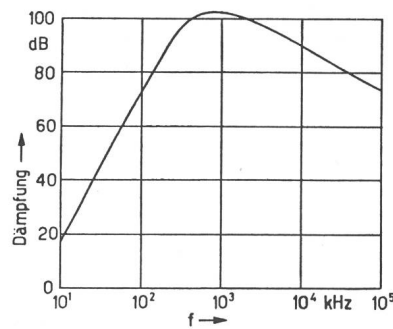
Fig. 7 Frequenzgang der Dämpfung eines kommerziellen Netzfilters
