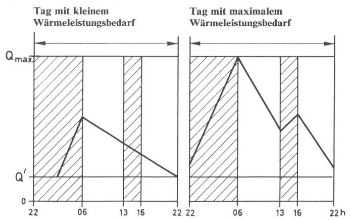
Fig. 5 Aufladeproduktionscharakteristik bei 3 Stunden Tagesnachladung
