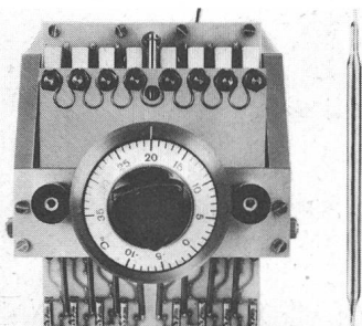
Kapillarrohrthermostat Typ Maxi-Multistat, 6 bis 8 Stufen
