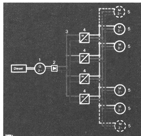
Fig. 9 Prinzipschaltbild der dieselektrischen Lokomotive DE 2500
