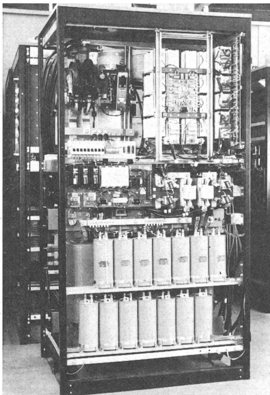
Fig. 8 USV-Anlage, Typ AGIETRONIC
