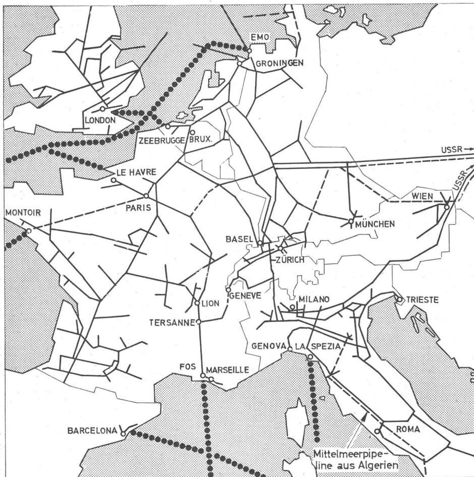
Fig. 3 Europäisches Erdgasverteilnetz
