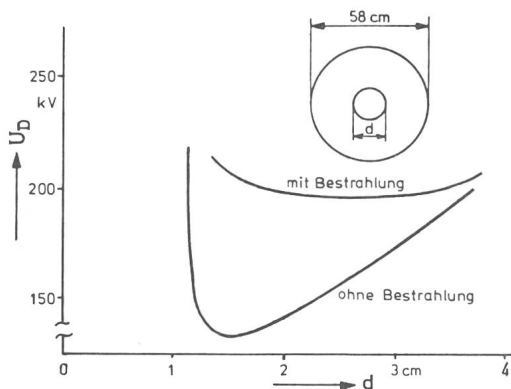
Fig. 2 Durchschlags spannung zwischen zwei koaxialen Zylindern in Abhängigkeit vom Durchmesser d des Innenleiters, ohne und mit Bestrahlung [15]
