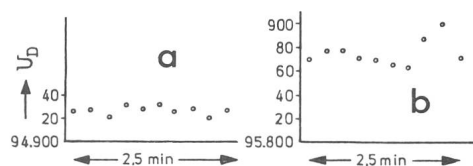
Fig. 5 Statische Durchschlagsspannung U_D bei aufeinanderfolgenden Durchschlägen in Stickstoff p = 7,8 bar, d = 0,5 cm, Wo-Elektroden [32] a UV-bestrahlt, b unbestrahlt
