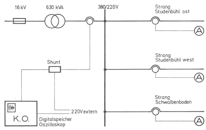
Fig. 6 Messeinrichtung Ipoliges Prinzipschema
