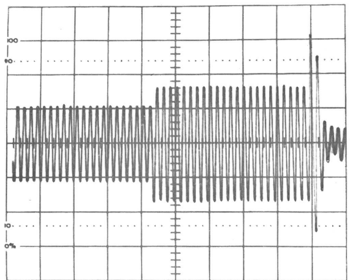
Fig. 2 x-Achse: 100 ms/div; y-Achse = 20 A/div Kompressor wie in Fig. 1 aber mit 2stufigem Anlasswiderstand 10/5 \Omega ohne Druckentlastung. Der Motor dreht erst nach dem Kurzschliessen der Anlasswiderstände I_1 = 16 A; I_2 = 24 A; I_A = 44 A; T_A = 950 ms
