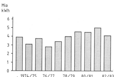
Fig. 6 Fremdenergiebezug
