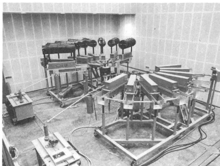
Fig. 6 Stossstromanlage am Institut für Elektrische Energieversorgung der Hochschule der Bundeswehr München
