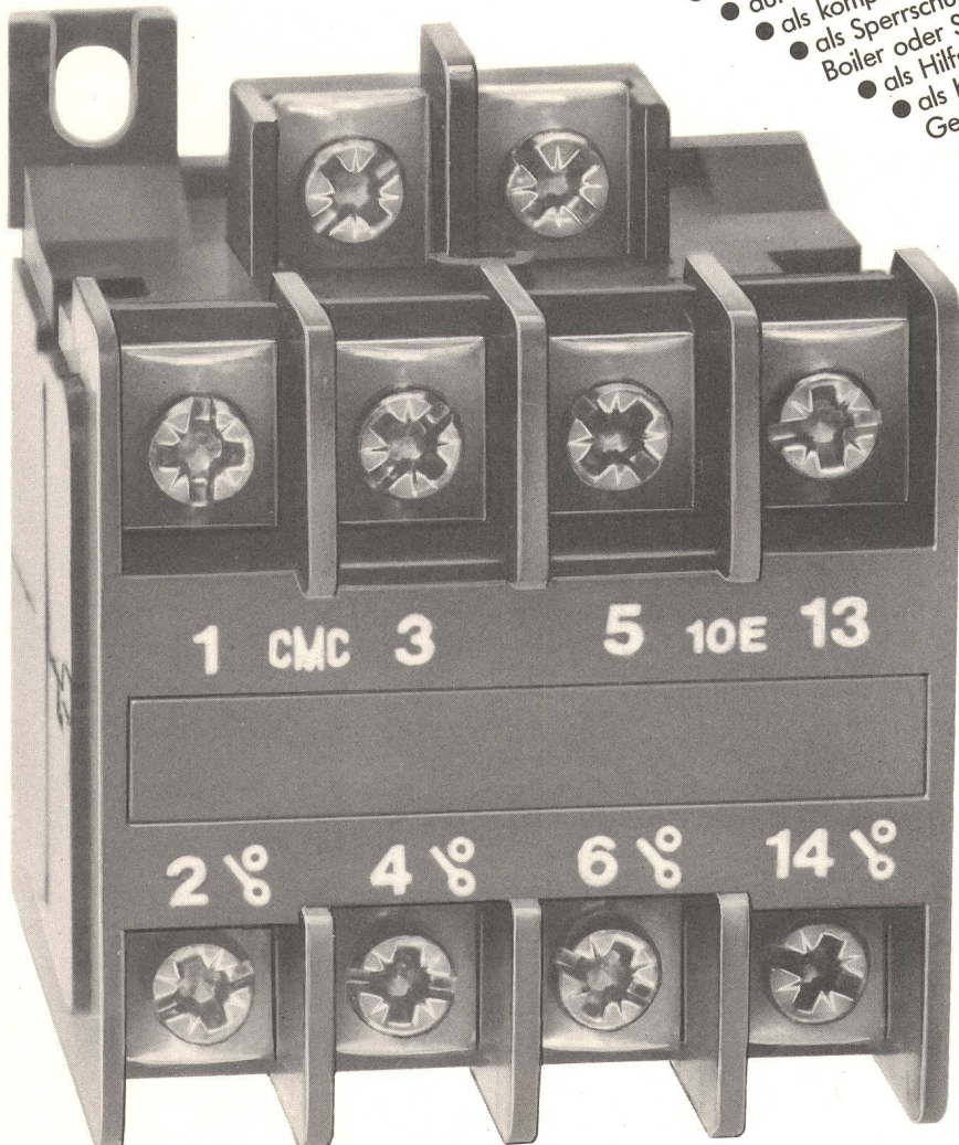
Originalgrösse 45 × 58 × 52 mm
