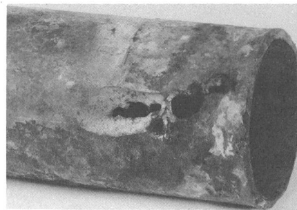
Fig. 3 Die korrodierte Guss-Wasserleitung
