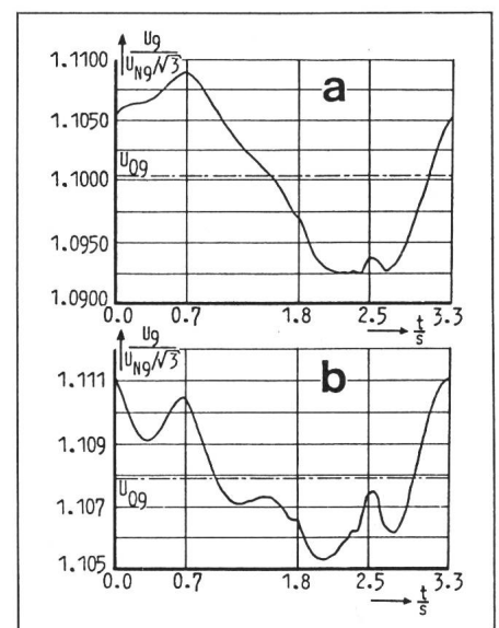
Fig. 2 Spannungsverlauf eines Generators im Netz des Synchro-Zyklotrons a Spannungsverlauf ohne Synchronphasenschieber b Spannungsverlauf mit Synchronphasenschieber
