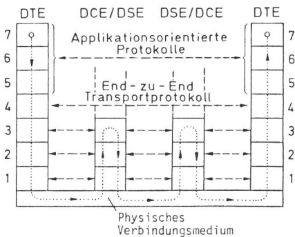
Fig. 8 OSI-Modell der ISO für offene Systeme
