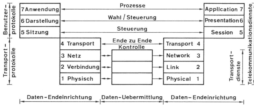
Fig. 1 OSI-Architektur-Modell
